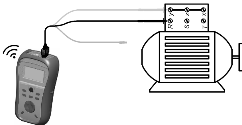
Figura 5.11: Applicazione del cavo di prova universale
