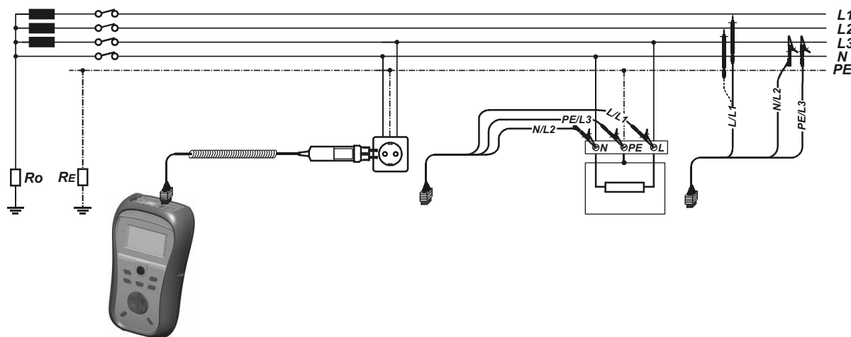
Afbeelding 5.27: Fase-neutraal of fase-fase lijnimpedantiemeting - aansluiting van stekkercommandant en universele testkabel
