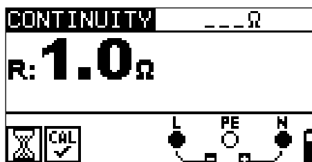
Figure 5.12: Exemple de mesure continue de la résistance
