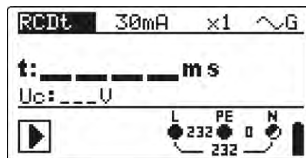
Rysunek 5.16: Test RCD
