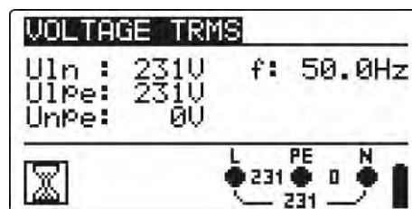
Rysunek 5.1: Napięcie w układzie jednofazowym
