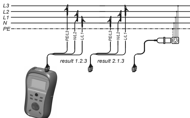
Figura 5.2: Collegamento del cavo di prova universale e dell'adattatore opzionale nel sistema trifase
