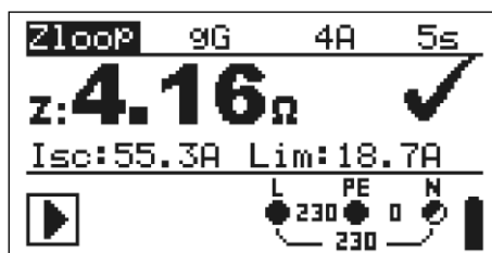
Afbeelding 5.25: Voorbeelden van meetresultaten lusimpedantie
