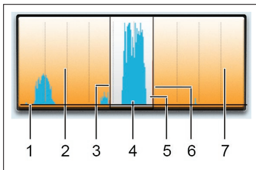
Fig. 21: Affichage de la fréquence 1 Axe de fréquence, 2 Bande non passante inférieure, 3 Limite de filtre inférieure, 4 Affichage graphique des fonctions, 5 Bande passante, 6 Limite de filtre supérieure, 7 Bandes non passante supérieure,
