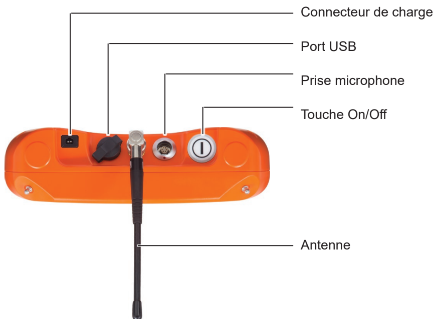
Fig. 2: Récepteur C 200, vue de dessus
