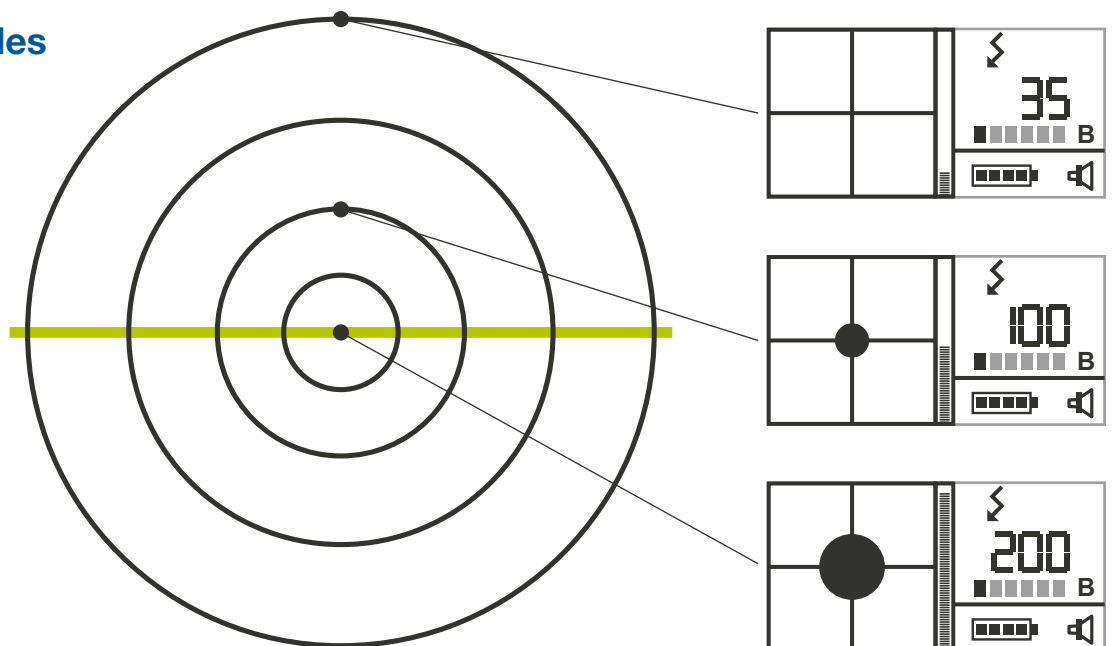
Affichage à l'écran lors de la localisation de câbles conducteurs
