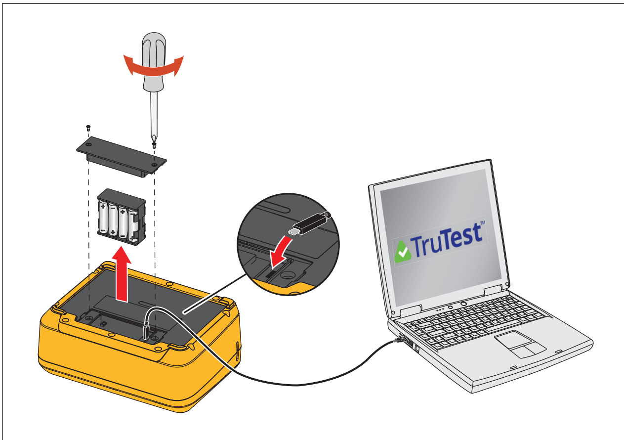
Afbeelding 24. Firmware updaten
