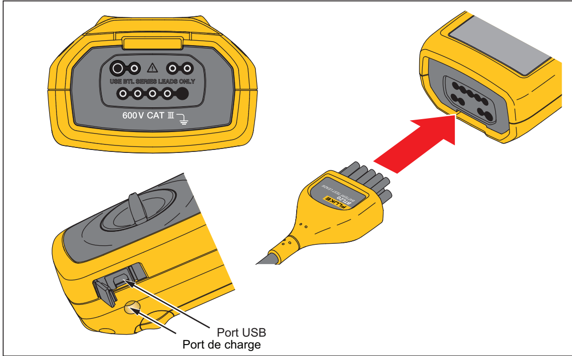
Figure 1-2. Bornes d'E/S
