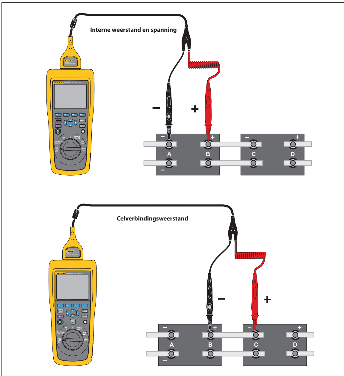
Figure 3-1. Test de la résistance interne et de la tension de la batterie ou de la résistance de la sangle
