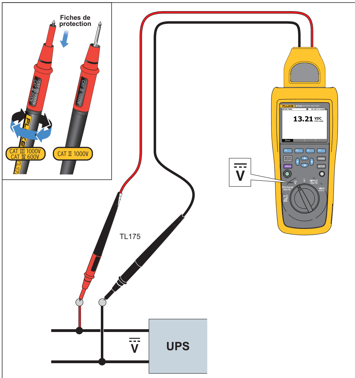
Figure 3-5. Mesure de la tension continue avec le TL175
