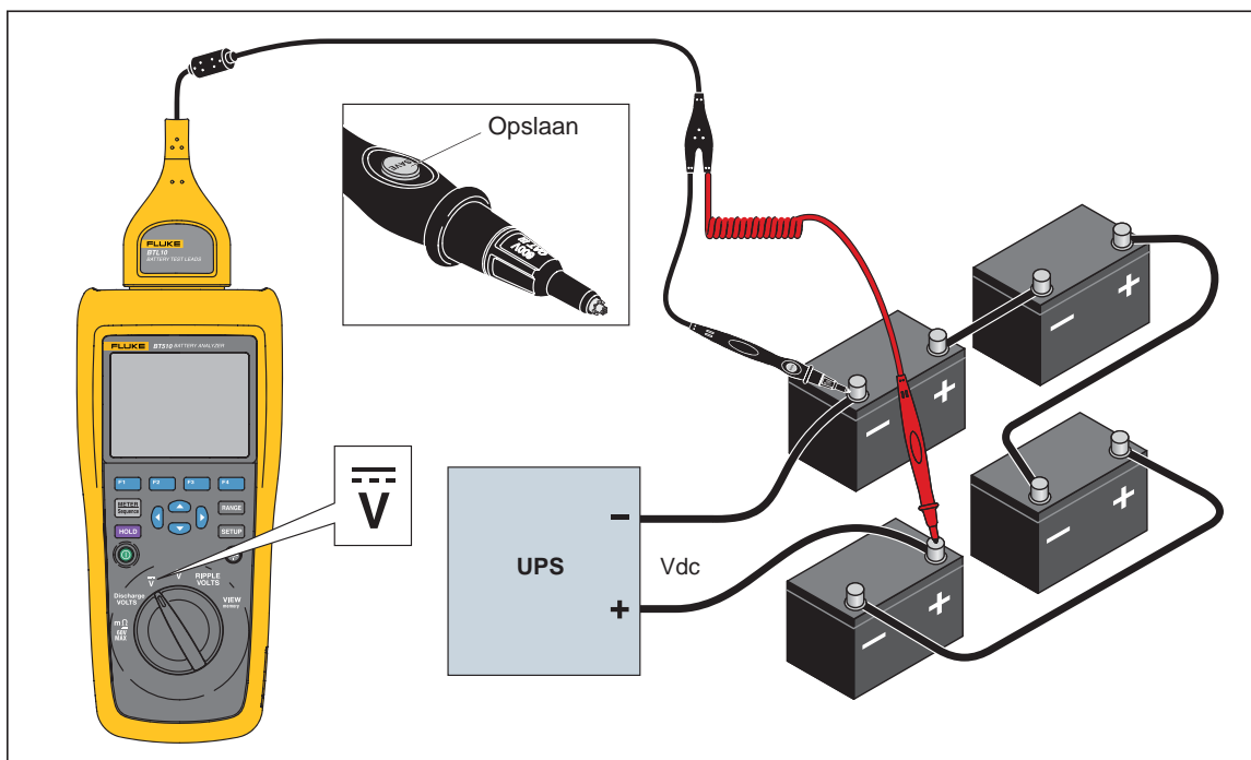
Afbeelding 3-3. DC-spanning meten
