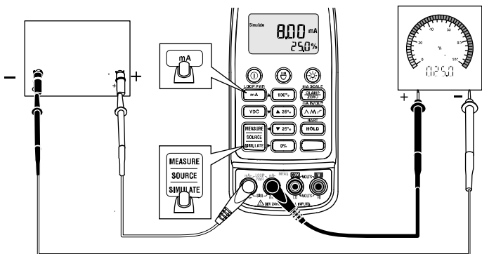
Afbeelding 9. mA-uitvoer simuleren
