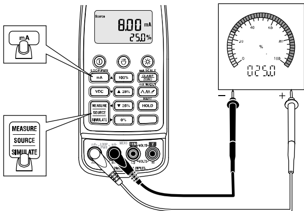
Afbeelding 8. mA-uitvoer aanvoeren
