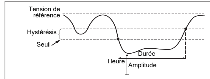
Figure 12. Caractéristiques d'un creux de tension
