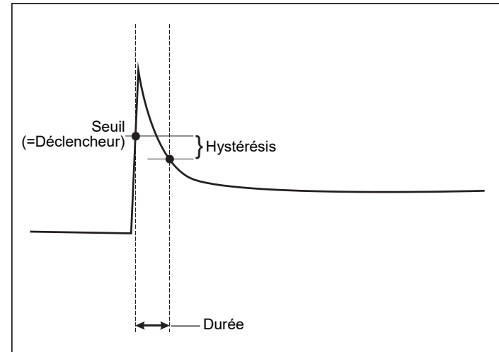
Figure 14. Caractéristiques du démarrage et rapport avec le menu de démarrage
