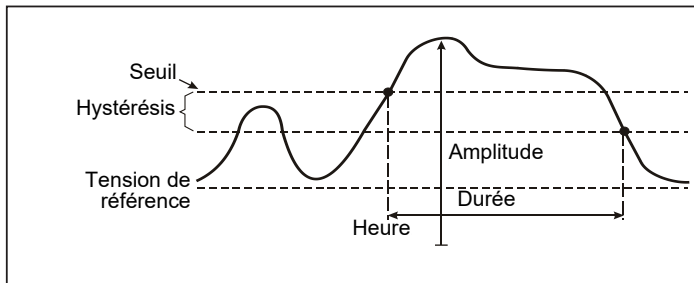
Figure 11. Caractéristiques d'une hausse de tension
