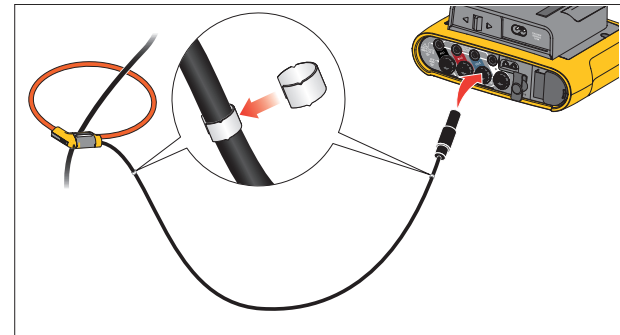
Figure 4. Cordons de mesure avec marqueurs de câbles
