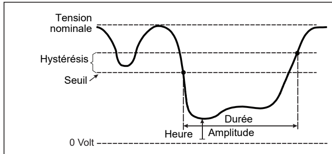
Figure 13. Caractéristiques d'une coupure de tension
