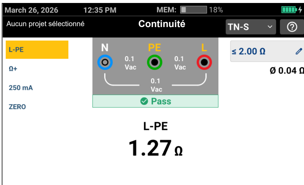
Figure 6. Affichage du zéro
