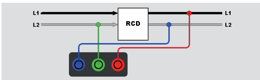
Figure 17. Connexion pour le test de différentiel de type B ou de différentiel de type A-EV sur les systèmes électriques IT
