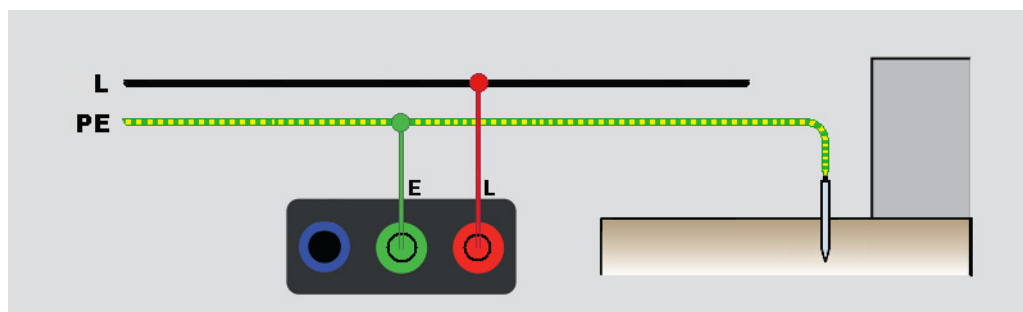
Figure 24. Raccordement à deux cordons pour le test de boucle de résistance de terre (courant de déclenchement élevé)
