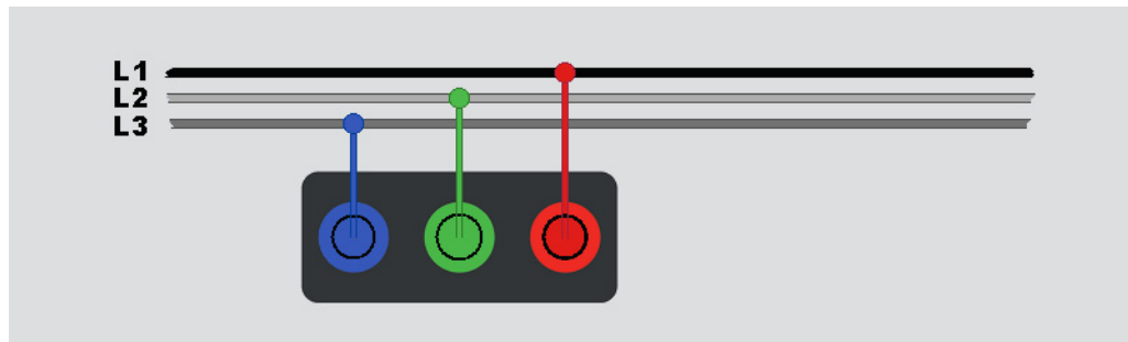
Figure 18. Raccordement de test de rotation de phase
