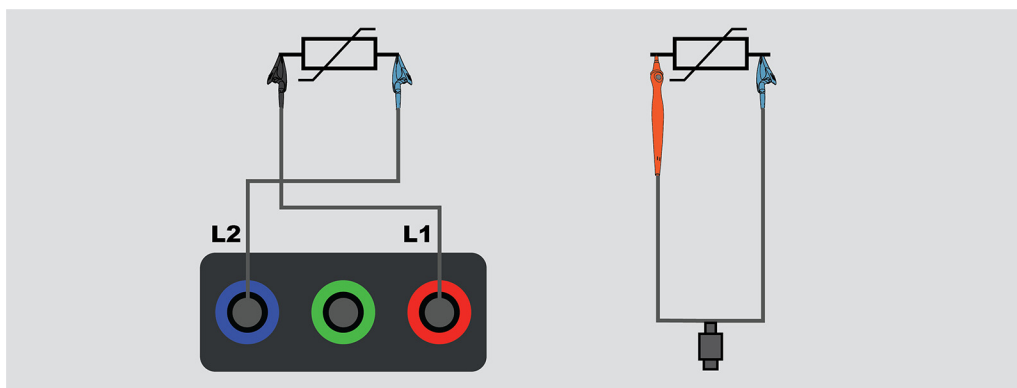
Figure 21. Connexion de test de SPD
