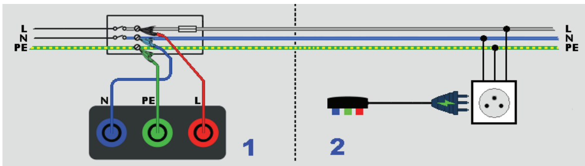
Figure 20. Connexion de test de chute de tension
