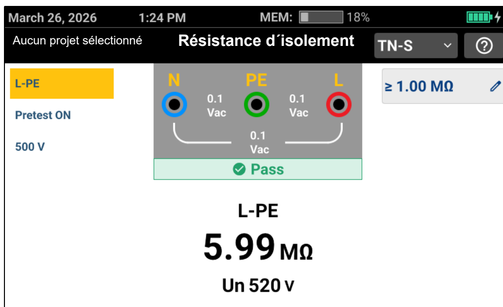
Figure 9. Ecran de mesure de résistance d'isolement
