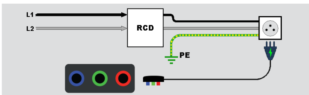
Figure 16. Configuration à cordon de mesure unique
