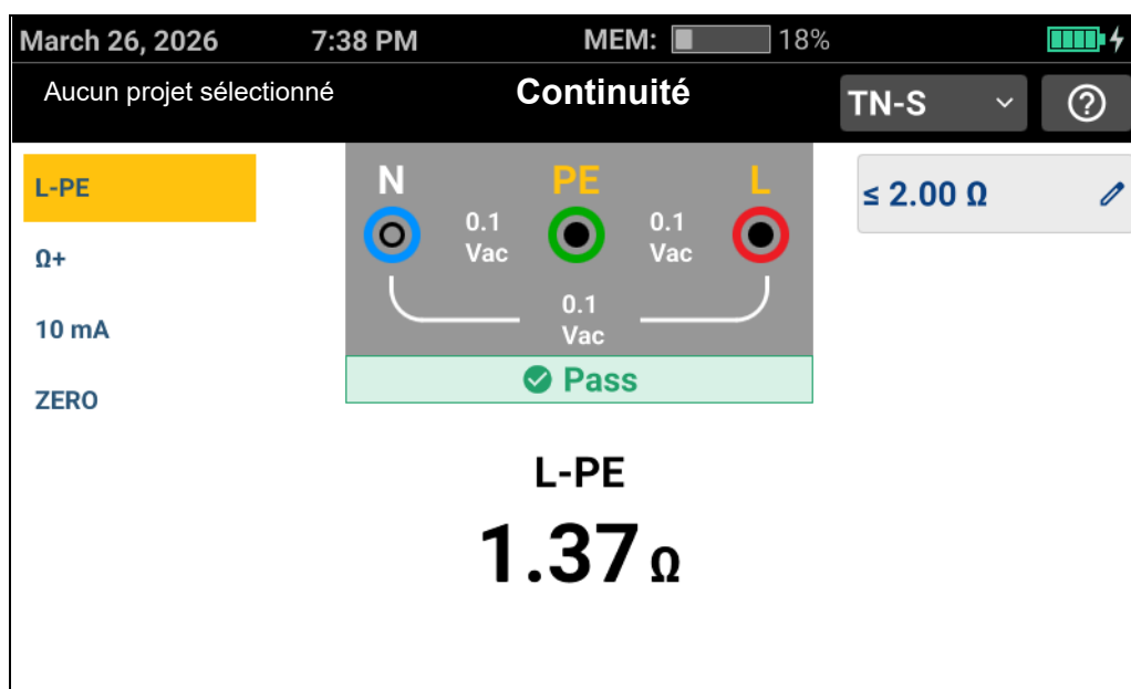
Figure 10. Ecran de mesure de continuité
