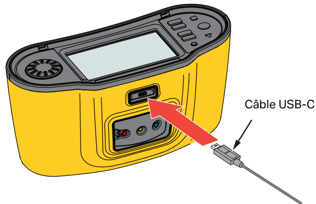
Figure 26. Connexion du câble USB-C
