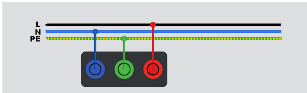
Figure 23. Raccordement à trois cordons pour le test de boucle de résistance de terre (mode sans déclenchement)
