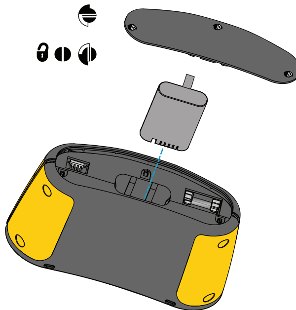
Figure 27. Remplacement des piles
