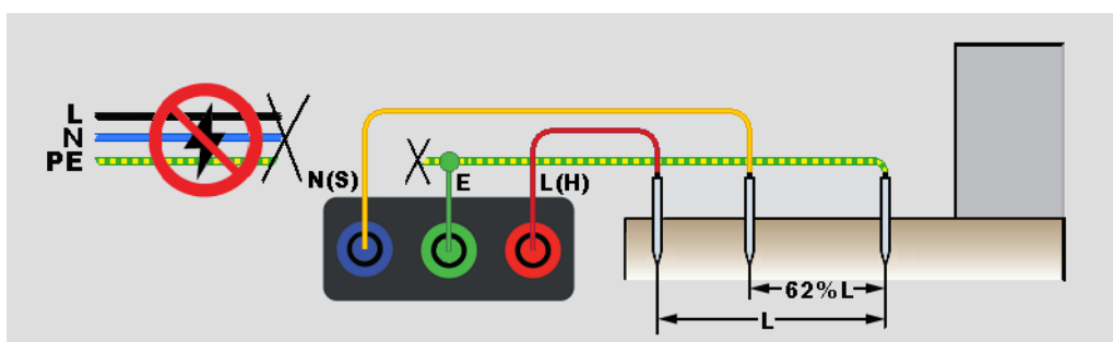
Figure 19. Raccordement de test de la résistance de terre
