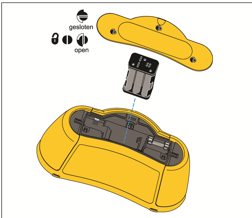
Afbeelding 20. Batterijen vervangen
