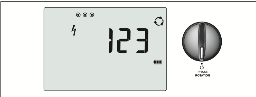
Afbeelding 14. Faserotatiedisplay
