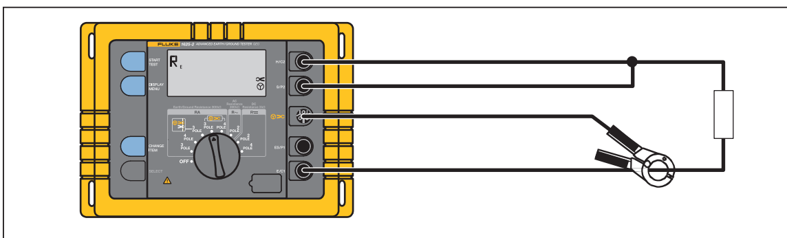
Afbeelding 9. Stroomtang/-transformator aansluiten
