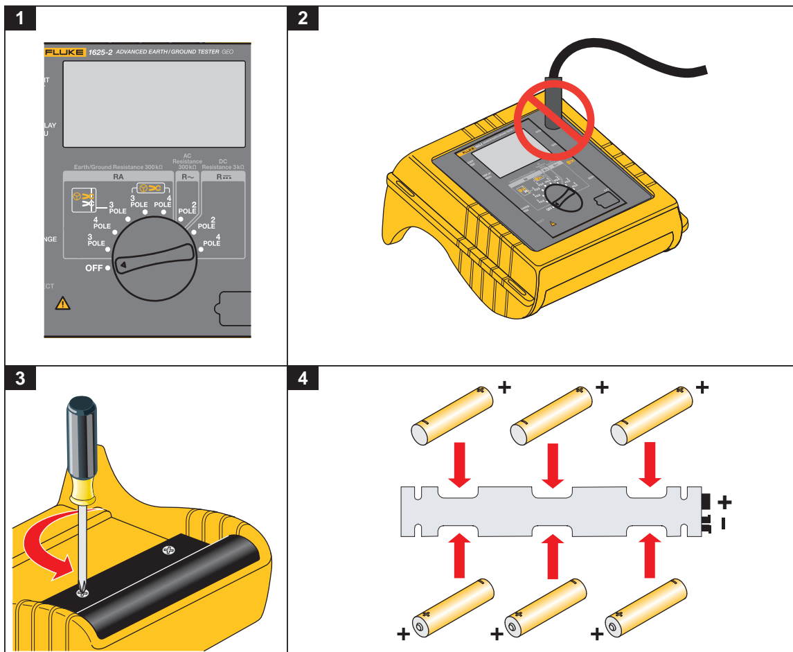
Afbeelding 2. Batterijen plaatsen
