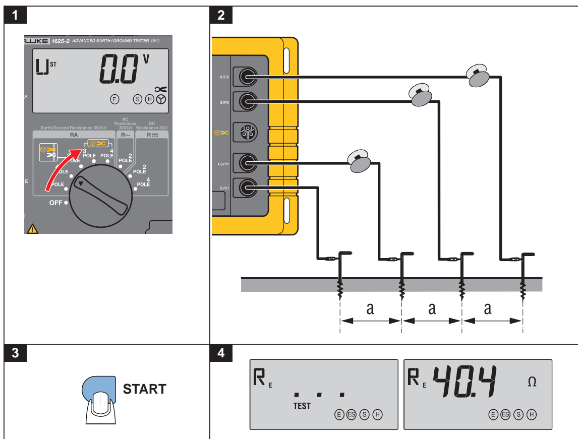
Abbeelding 11. Meting van bodemweerstand
