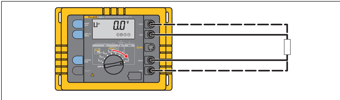
Afbeelding 13. Weerstandsmeting ( R_{\text{---}} )
