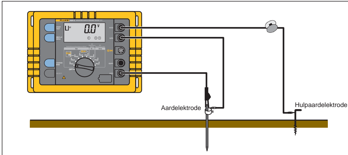
Afbeelding 10. Compensatie van de weerstand van het op de aardelektrode aangesloten snoer
