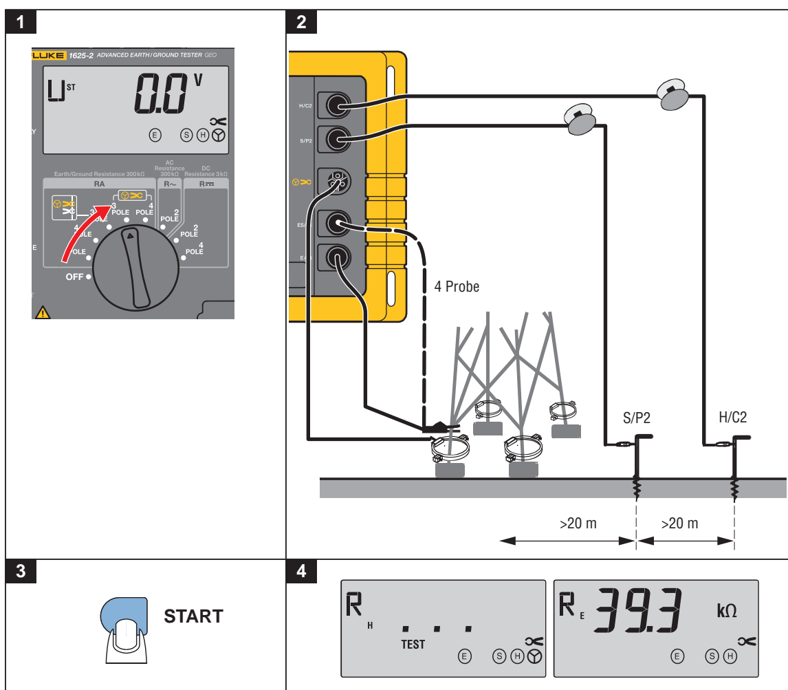
Afbeelding 7. Aardingsweerstand zonder loskoppeling van de bliksemdraad
