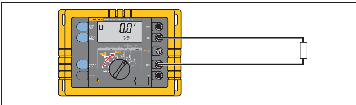
Afbeelding 12. Weerstandsmeting ( R\sim )
