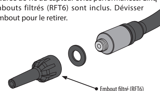
Embout filtré (RFT6)
