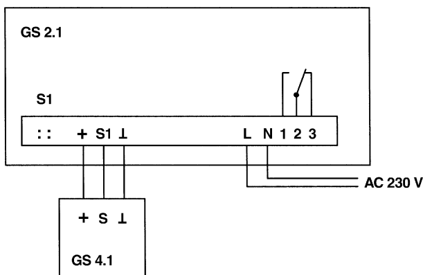
Figure 4 : Branchement électrique GS 2.1 et GS 4.1. Relais représenté sans courant = situation d'alarme
