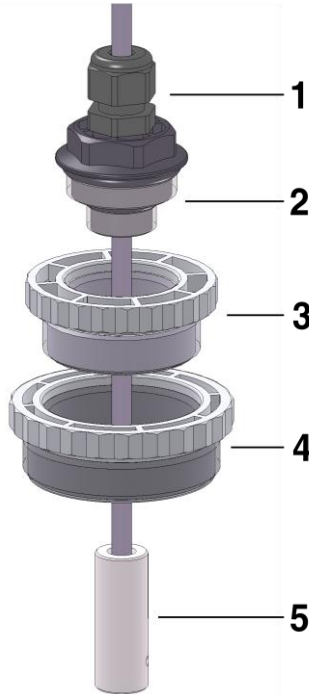
Fig. 6 : Montage sur le réservoir avec set de raccords à vis
