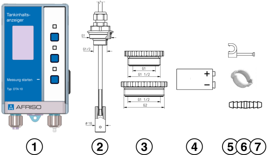
Fig. 1 : Étendue de la livraison de l'indicateur numérique de niveau de réservoir DTA 10
