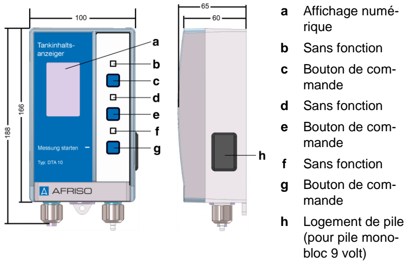
Fig. 3 : Appareil de mesure (dimensions en mm)
