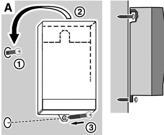
Fig. 5 : Fixation de l'appareil de mesure
